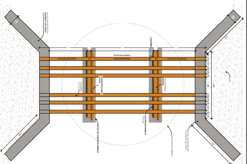
2 LONGARINAS Escala: 1 : 50
