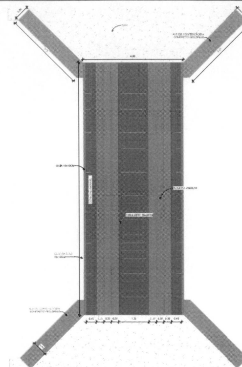
3 PISO DA PONTE Escala 1:50
